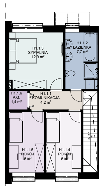
PIĘTRO
